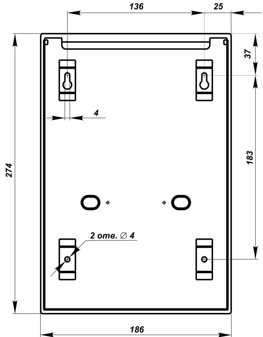
Приложение Г Установочные и габаритные размеры прибора (вид со стороны крепления)
