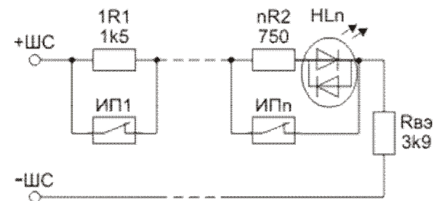
Рисунок 4 – Схема включения пассивных извещателей с размыкающимися контактами типа «МАК-1» (исп. 01 ИБ, исп. 011 ИБ) для формирования извещения «Внимание».
