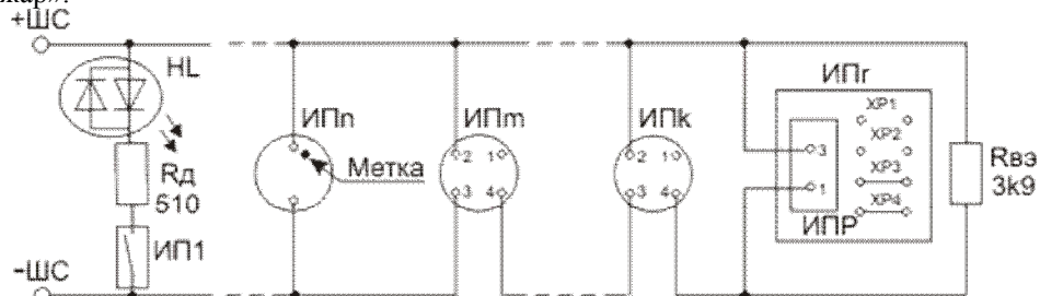
Рисунок 2 – Схема включения пассивного извещателя с замыкающимися контактом типа «МАК-1» исп. 011 ИБ и токопотребляющих извещателей типа «МАК-ДМ» ИБ исп. 01, «ИД(Т)-2» ИБ, «УФИС» ИБ, ИПР «АГАТ» ИБ для формирования извещения «Пожар».
