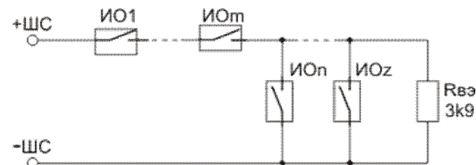
Рисунок 5 – Схема включения охранных извещателей для формирования извещения «Проникновение».
