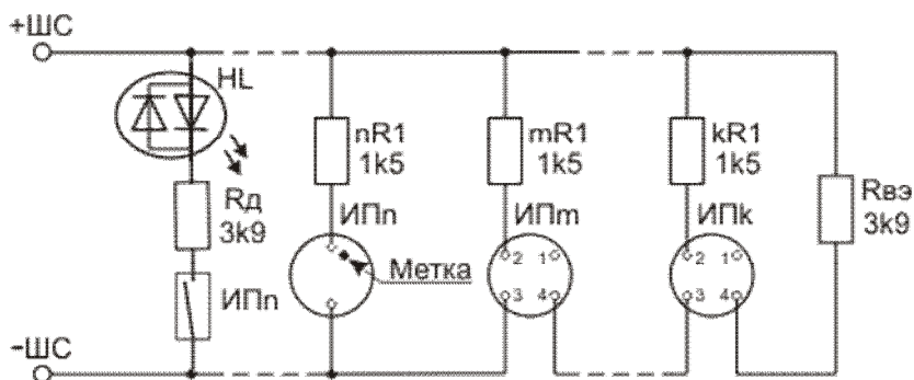
Рисунок 3 – Схема включения пассивного извещателя с замыкающимися контактом типа «МАК-1» исп. 011 ИБ и токопотребляющих извещателей типа «МАК-ДМ» ИБ исп. 01, «ИД(Т)-2» ИБ, «УФИС» ИБ для формирования извещения «Внимание».
