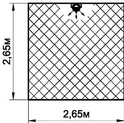
Рисунок 7 - Масштабное изображение области, в которой достигаются условия тушения модулем Буран-2,0(1) по очагам класса В.
