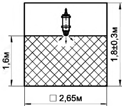
Рисунок 7 - Масштабное изображение области, в которой достигаются условия тушения модулем Буран-2,0(1) по очагам класса В.
