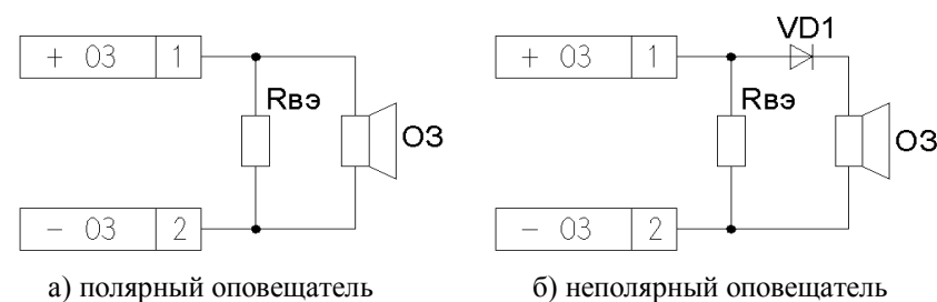
Рисунок Г.2 Схема подключения звукового оповещателя Rвэ – С1-4-0,25-1,2 кОм±5% VD1- диод 1N5400
