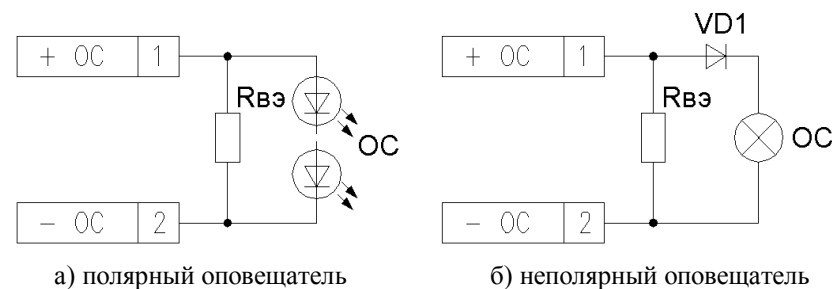
Рисунок Г.1 Схема подключения светового оповещателя Rвэ – С1-4-0,25-1,2 кОм±5% VD1- диод 1N5400
