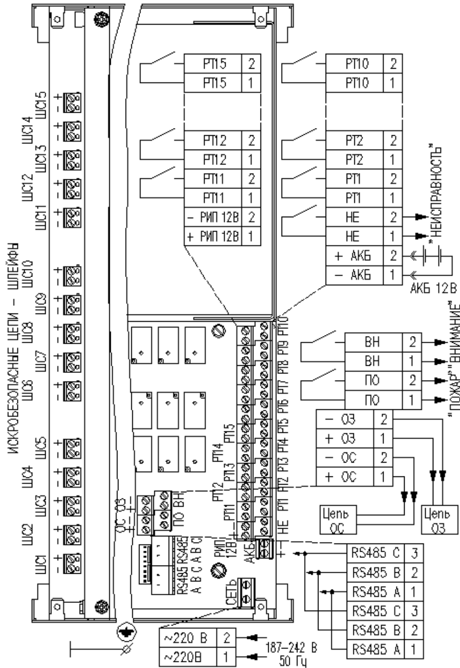
Рисунок А.3 Схема подключения прибора Корунд-20 СИ исп.-02 (15 ШС)
