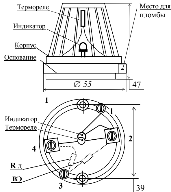
Рис. 1. Габаритные и установочные размеры, общий вид и расположение элементов в корпусе извещателя с замыкающимся контактом
