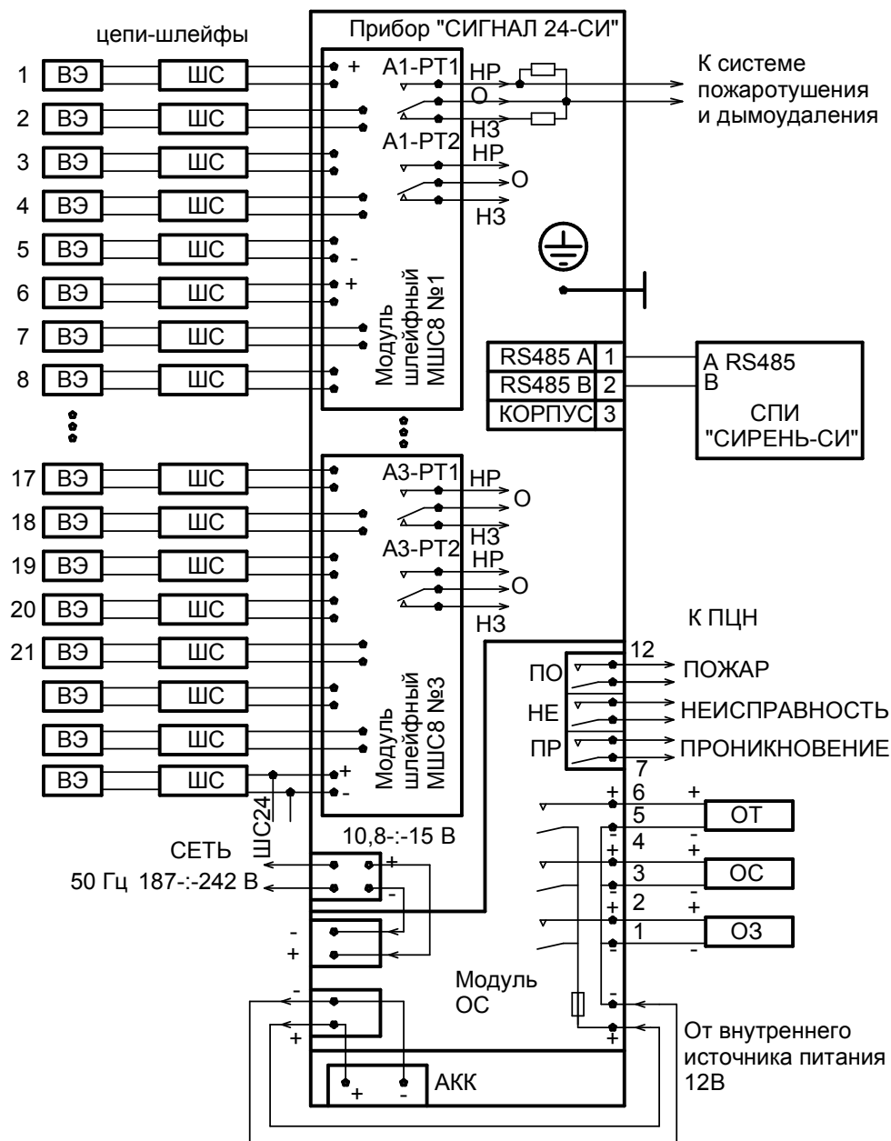
Приложение А Схема внешних соединений прибора
