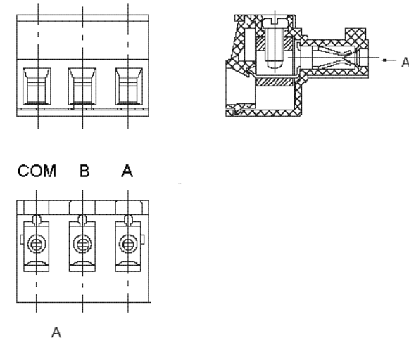
Внешний вид соединителя на кабеле связи по интерфейсу RS-485 Маркировка контактов на кабельной розетке
