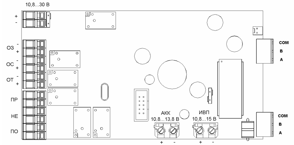
Внешний вид модуля обработки сигналов МОС Маркировка релейных выходов ПО, НЕ, ПР, выходов для питания внешних оповещателей ОТ, ОС, ОЗ, входов для подключения питания.
